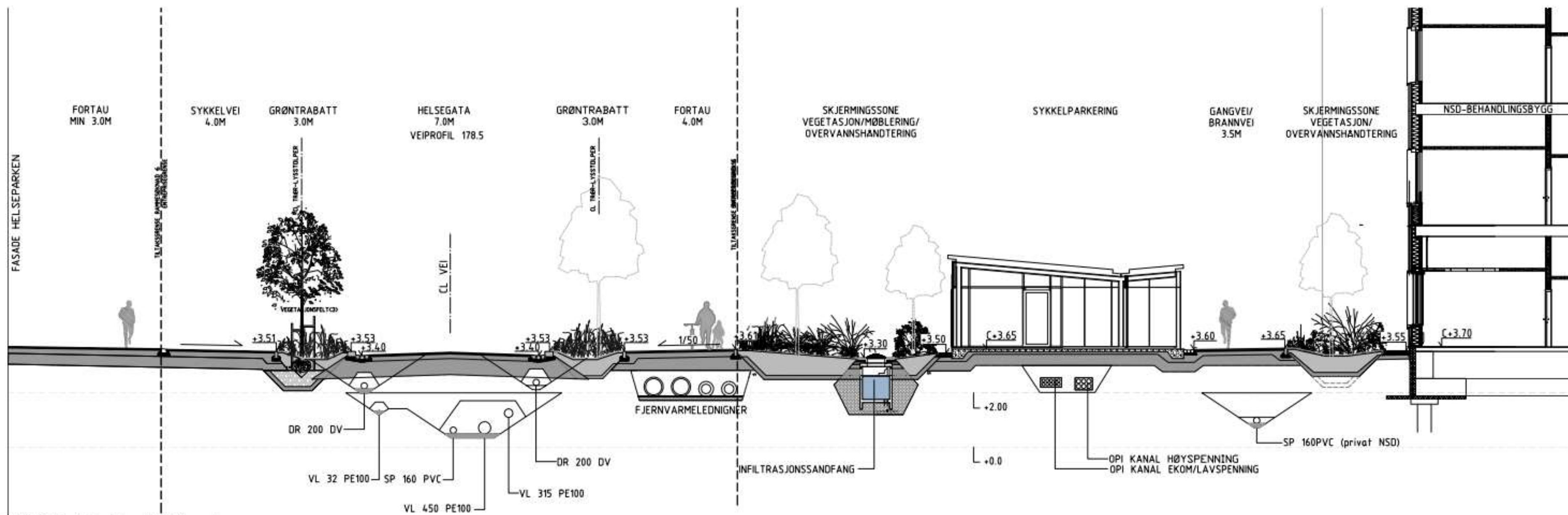
1 Snitt D-D - Teknisk snitt Helsegata Målestokk 1:100(A1)
